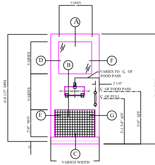
TYP. DOOR ELEVATION
