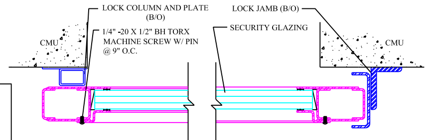
D TYP. DOOR DETAIL
