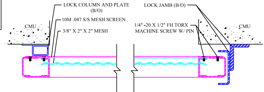
E TYP. DOOR DETAIL
