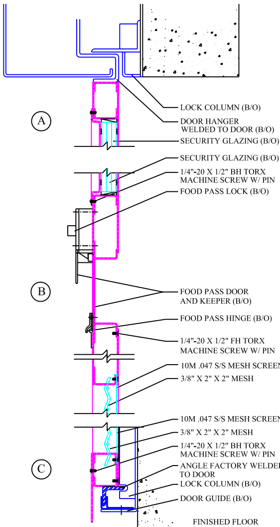
TYP. DOOR SECTION
