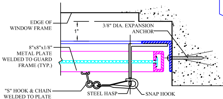
(D) TYP. JAMB DETAIL @ LOCK
